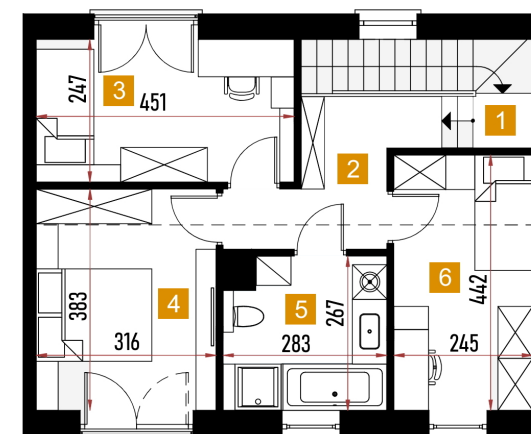
rzut piętra
