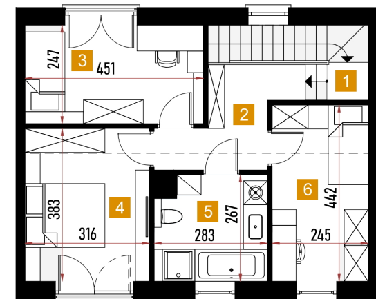
rzut piętra
