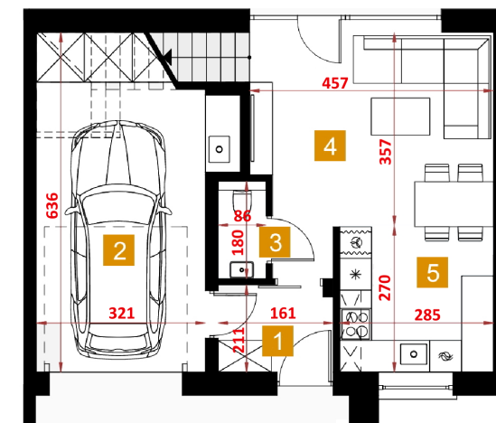
rzut parteru
