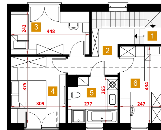
rzut piętra
