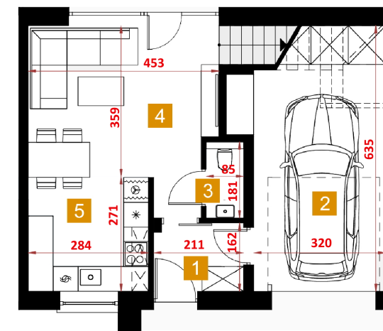
rzut parteru
