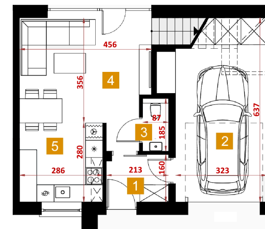
rzut parteru
